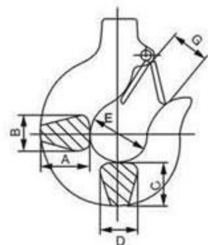
Hook 吊钩
